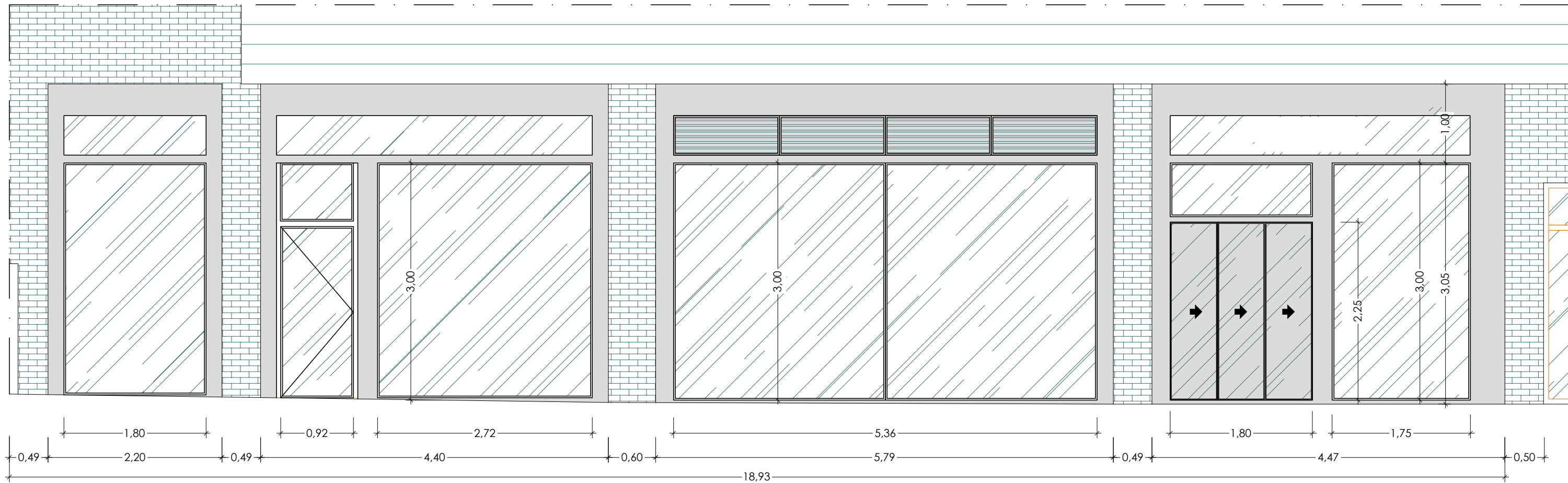
ALZADO DE FACHADA
